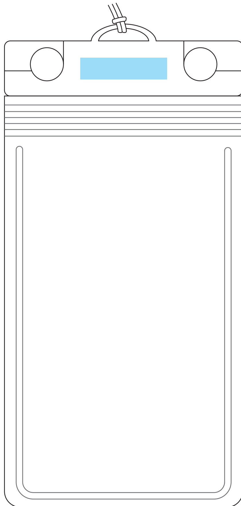
蓋 表面：W40×H10mm
