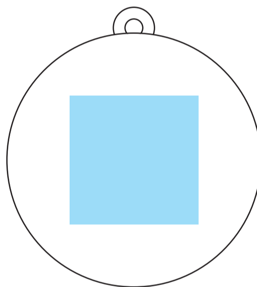
フタ天面 B : W35×H35mm
